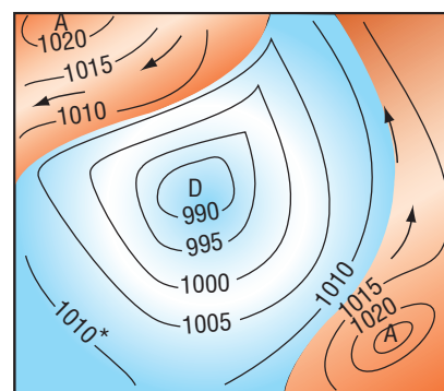
(D) : Depression (A) : Anticyclone
